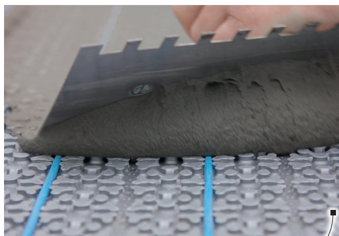
Natte à excroissances avec sous-face en non-tissé équipée de la technologie Grip Lock.
