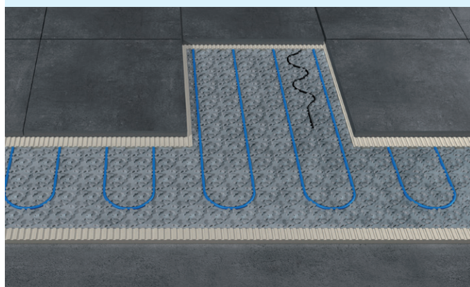
Natte à excroissances avec sous-face en non-tissé équipée de la technologie Grip Lock.
